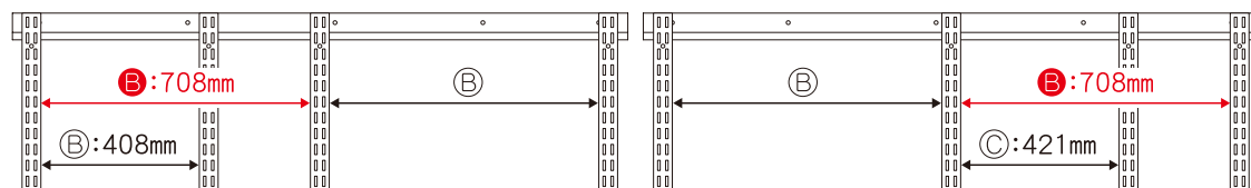
(棚板2枚連結)
