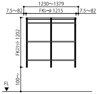
FKスリット 1202 2列 600+600 PLAN MC412a
