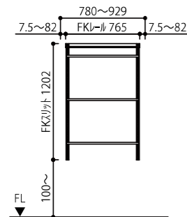
FKスリット 1202 1列 750 PLAN MC312a
