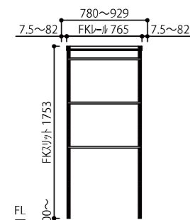
FKスリット 1753 1列 750 PLAN MC317a
