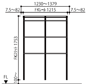
FKスリット 1753 2列 600+600 PLAN MC417a
