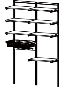
2列 600+600 PLAN MC419f
