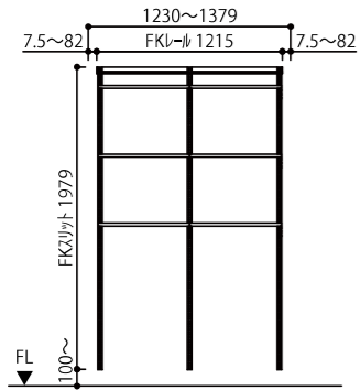
FKスリット 1979 2列 600+600 PLAN MC419a
