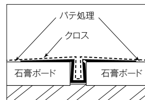
●施工例 内装ハット3mm
