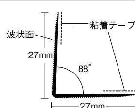
⑮ シャープコーナー 27
