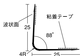
③ DX-4Rコーナー 25
