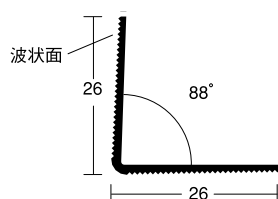
26 GLコーナー PA26
