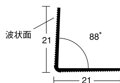
22 GLコーナー 21
