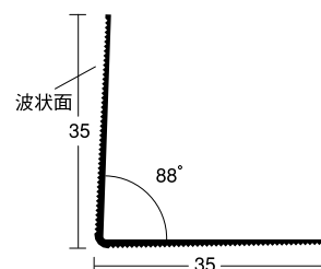
27 GLコーナー PA35
