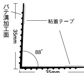
シャープエッジコーナー 35
