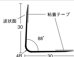
⑯ シャープ4Rコーナー
