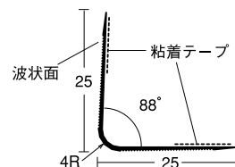
③ DX-4Rコーナー PA25®
