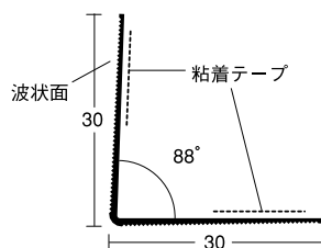
④ DX-KPコーナー 30 R
