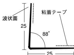
② DX-Kコーナー 25
