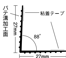
シャープエッジコーナー 27
