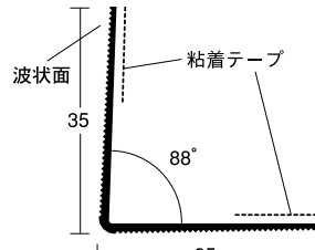
⑥ DX-KPコーナー 35
