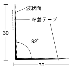
⑤ DX-KP入隅コーナー 30
