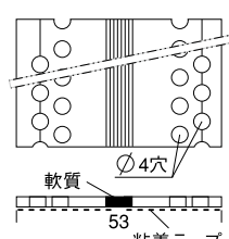
㉒ DX-ピタット4Rコーナー (2段パンチ穴)
