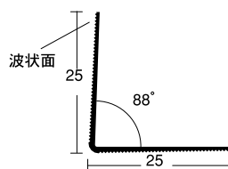
① KPコーナー 25
