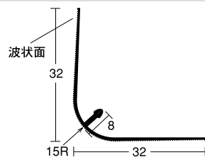
⑬ 15Rコーナー 32 (足付)
