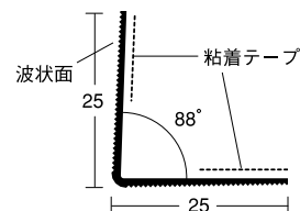
24 DXコーナーアングル25 ® (薄型)
