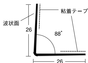
26 DX-GLコーナー PA26 ®
