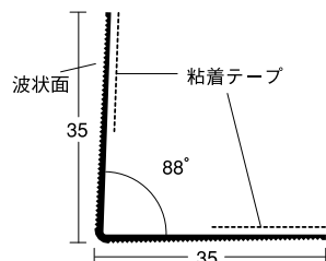
28 DX-GLコーナー PA35 ®
