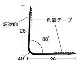
⑦ DX-KP4Rコーナー 26 R
