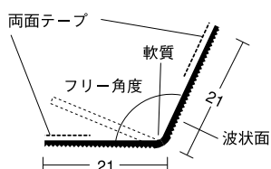
⑤ DXフリーコーナーライン21
