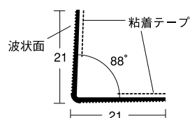
23 DX-GLコーナー 21
