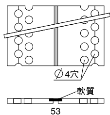
⑱ ピタットコーナー® (2段パンチ穴)
