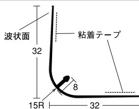
⑭ DX-15Rコーナー 32 (足付)
