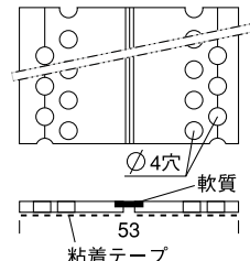
⑲ DX-ピタットコーナー® (2段パンチ穴)
