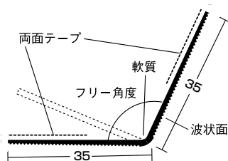
⑪ DX-KPフリーコーナー 35 (出隅・入隅兼用)
