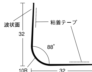
⑫ DX-10Rコーナー 32
