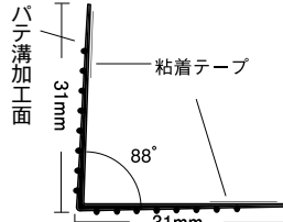
シャープエッジコーナー 31
