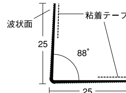
③ DX-KPコーナー 25 R
