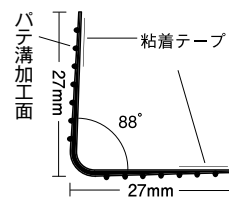
シャープエッジ4Rコーナー 27
