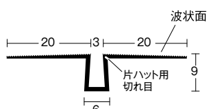
内装ハット3mm
