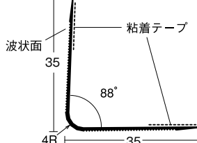
⑧ DX-KP4Rコーナー 35 R
